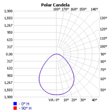
Misma luminaria con control de deslumbramiento WhiteOptics (DLC 5.1 Premium UGR)
