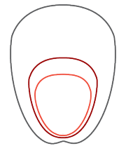
Medium Narrow Flood (MNFL) 60° de inclinación
